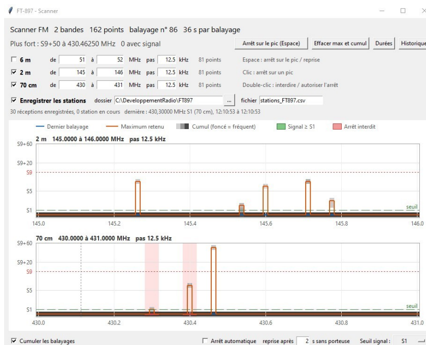
Figure 1. L'affichage de deux bandes et des fréquences reçues. La troisième bande n'est pas utilisée : elle n'est donc pas cochée.
